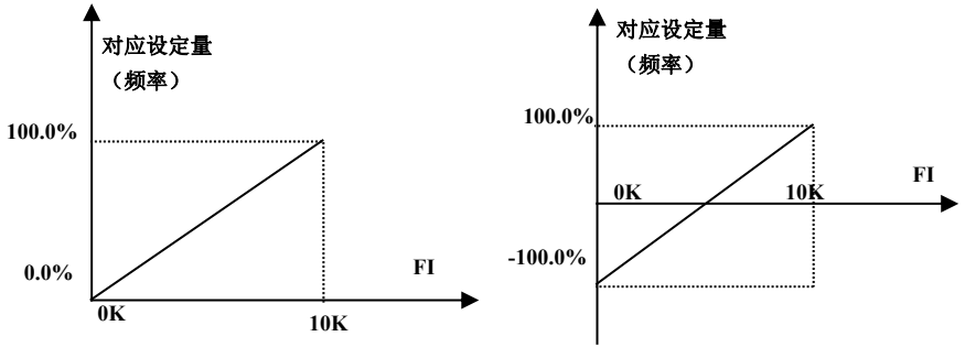
图 6-15 脉冲输入与设定量的对应关系
