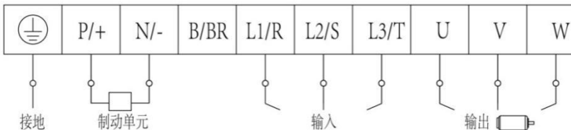
图 4-5 端子示意图
