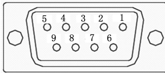
图 4-7 旋转变压器编码器端子排列示意图
