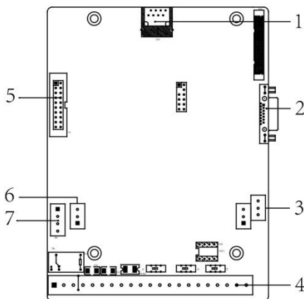
图 2-8 E7 及铁壳接口图
