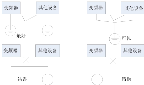
图 4-18 接地示意图
