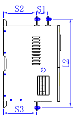
RC2 铜排结构尺寸
