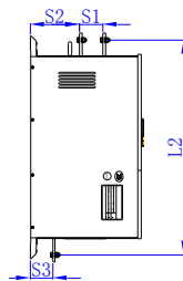
RC4 铜排结构尺寸
