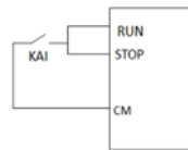
两线式
