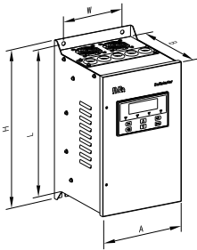
RC1 外形结构示意图
